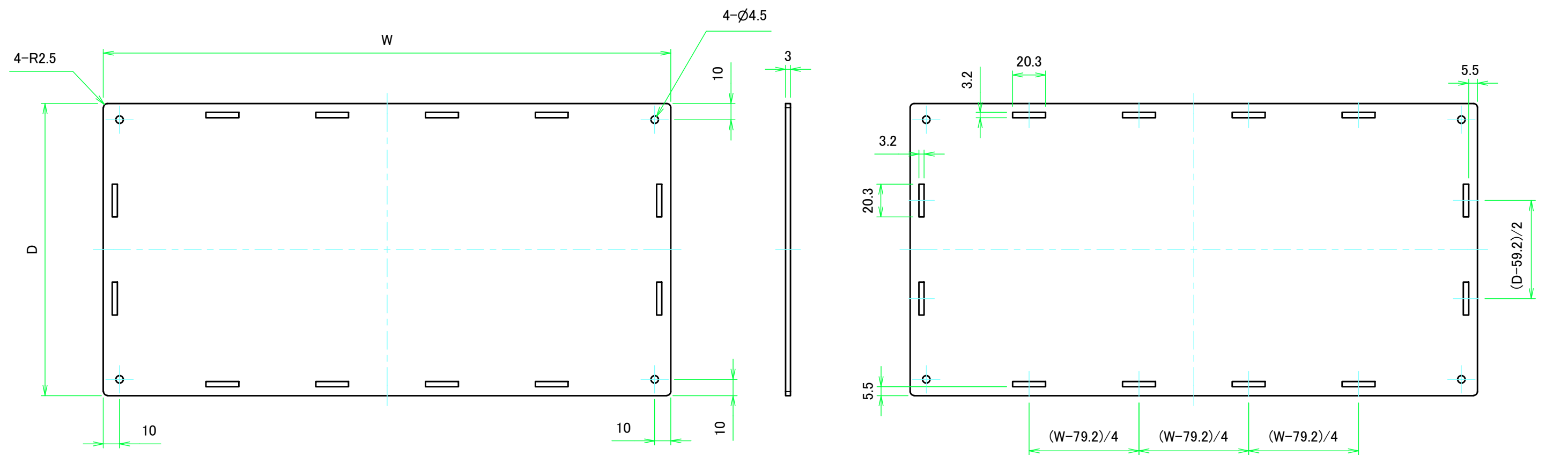
上カバー表面 / Top cover Frontside
