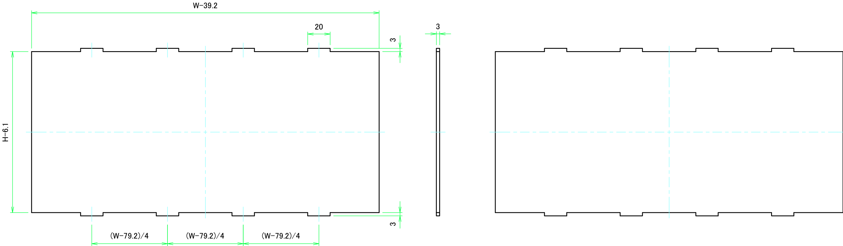
Wパネル1表面 / W Panel 1 Frontside
